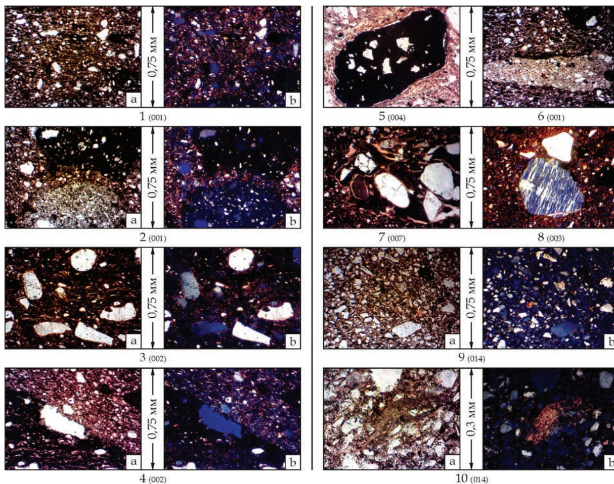
Рис. 6. Мікрофотографії шліфів кераміки: а, без літери — в просвічуючому поляризованому світлі, один поляризатор; б — в просвічуючому поляризованому світлі, схрещені поляризатори; 1 — формувальна маса петрогрупи 1 (ГС 1); 2 — керамокласти першого і другого типів у формувальній масі петрогрупи 1; 3 — формувальна маса петрогрупи 1 (ГС 2); 4 — шамот із ГС 1 (права верхня частина зображення) контактує з матрицею із ГС 2 (ліва нижня частина зображення); 5–7 — керамокласти першого, другого і третього типів у петрогрупі 1; 8 — включення із пертитовим зростанням; 9 — формувальна маса експериментального брикету з глинистої сировини; 10а–11б — звітрений біотит у формувальній масі експериментального брикету (в дужках вказано номер зразка)
