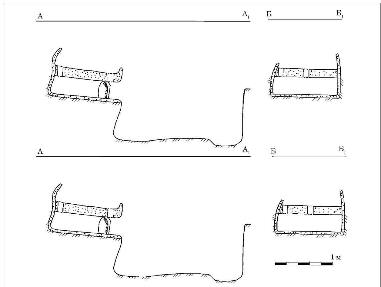
Рис. 7. Рукомиш II: гончарна майстерня, перерізи. Позначки див на рис. 5
