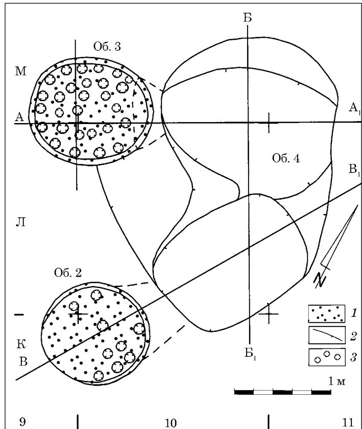
Рис. 6. Рукомиш II. План гончарної майстерні: 1 — гончарні горни; 2 — контури майстерні; 3 — продухи
