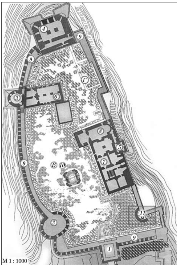
Рис. 2. Генеральний план замку Хотинської фортеці з місцем розташування Південно-східної башти: 1 — Південна (Візна) башта; 2 — Південно-західна башта; 3 — Західна (Комендантська) башта; 4 — Північна башта; 5 — Східна вежа; 6 — Комендантський палац; 7 — Казарма; 8 — Замкова церква; 9 — Оборонні мурів замку; 10 — Замкова криниця; 11 — залишки Південно-східної башти; В — двір воїнів; Г — княжий двір
