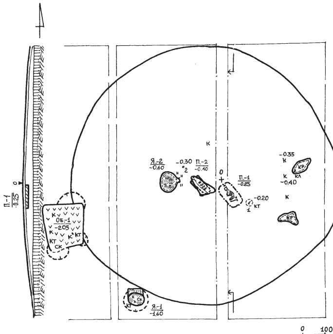
Рис. 1. Єристівка, с. Група II, курган № 2. План і східний профіль центральної бровки.
