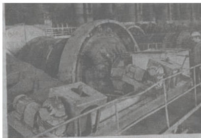
Колетива Дніпровського гірничо-збагачувального заводу успішно виконала взяті наперед'їздові зобов'язання, видавши близько двадцяти тисяч тонн концентрату руди. На фото: млиновий проліт збагачувальної фабрики руди перетворюється в порошок. Фото П. Кекала. (Фотохроніка РГТАЗ)
