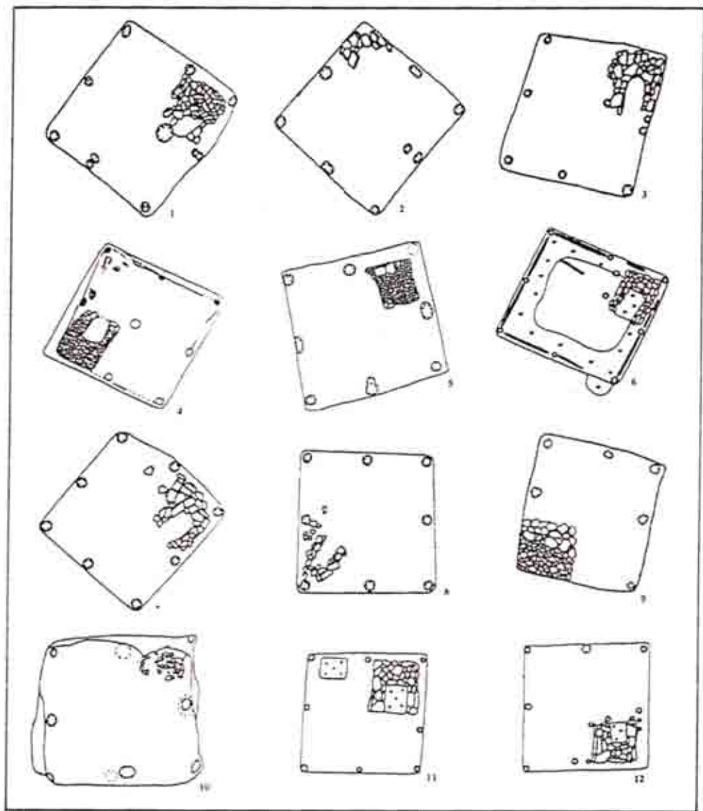
Рис. 38. Житла-напівземлянки першого варіанту стовпової конструкції.
