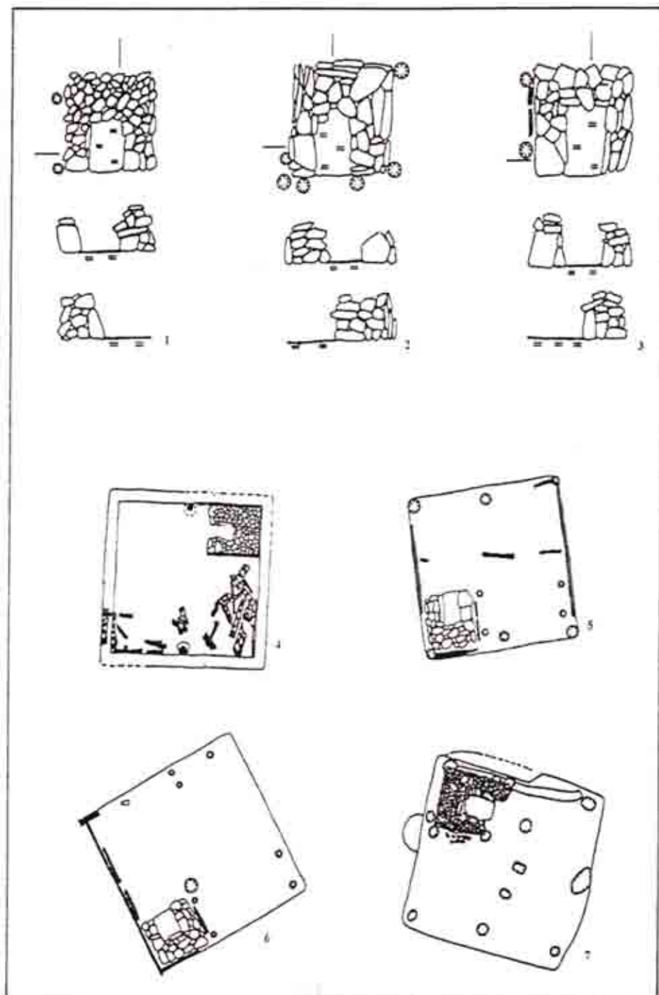
Рис. 44. Печі-кам'янки із слідами дере'яних конструкцій.
