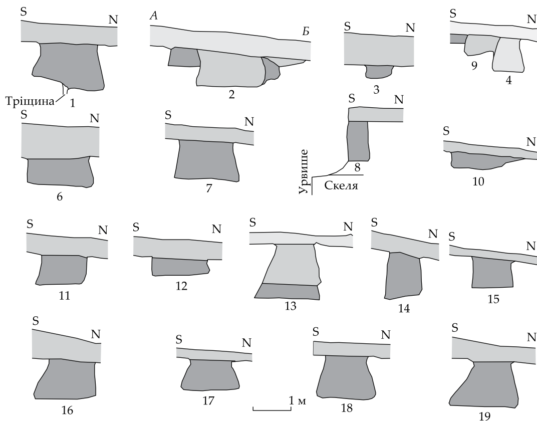
Рис. 13. Схеми профілів і проекцій ям розкопу 2 поселення Уч-Баш та стратиграфічних розрізів (за Є.О. Жеребцовим, 1953, НА НЗХТ, д. 690/Па). Цифрами позначено номери ям
