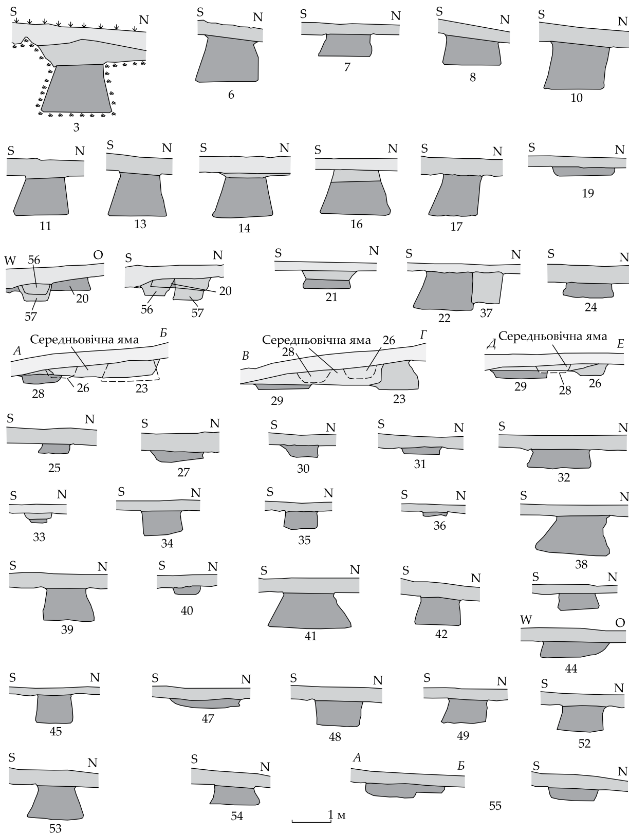
Рис. 5. Схеми профілів і проєкцій ям розкопу 1 поселення Уч-Баш та стратиграфічних розрізів (за Є.О. Жеребцовим, 1953, НА НЗХТ, д. 690/Па). Цифрами позначено номери ям
