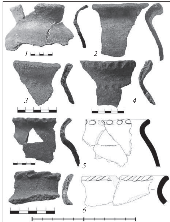
Рис. 5. Горшки з горлом у вигляді розтрубу, ділянка Г (2012—2017 pp.)
