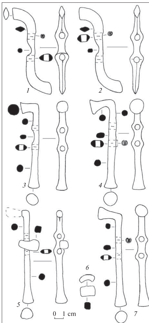
Рис. 10. Бронзові псалії з фрагментами залізних вудил з могили
