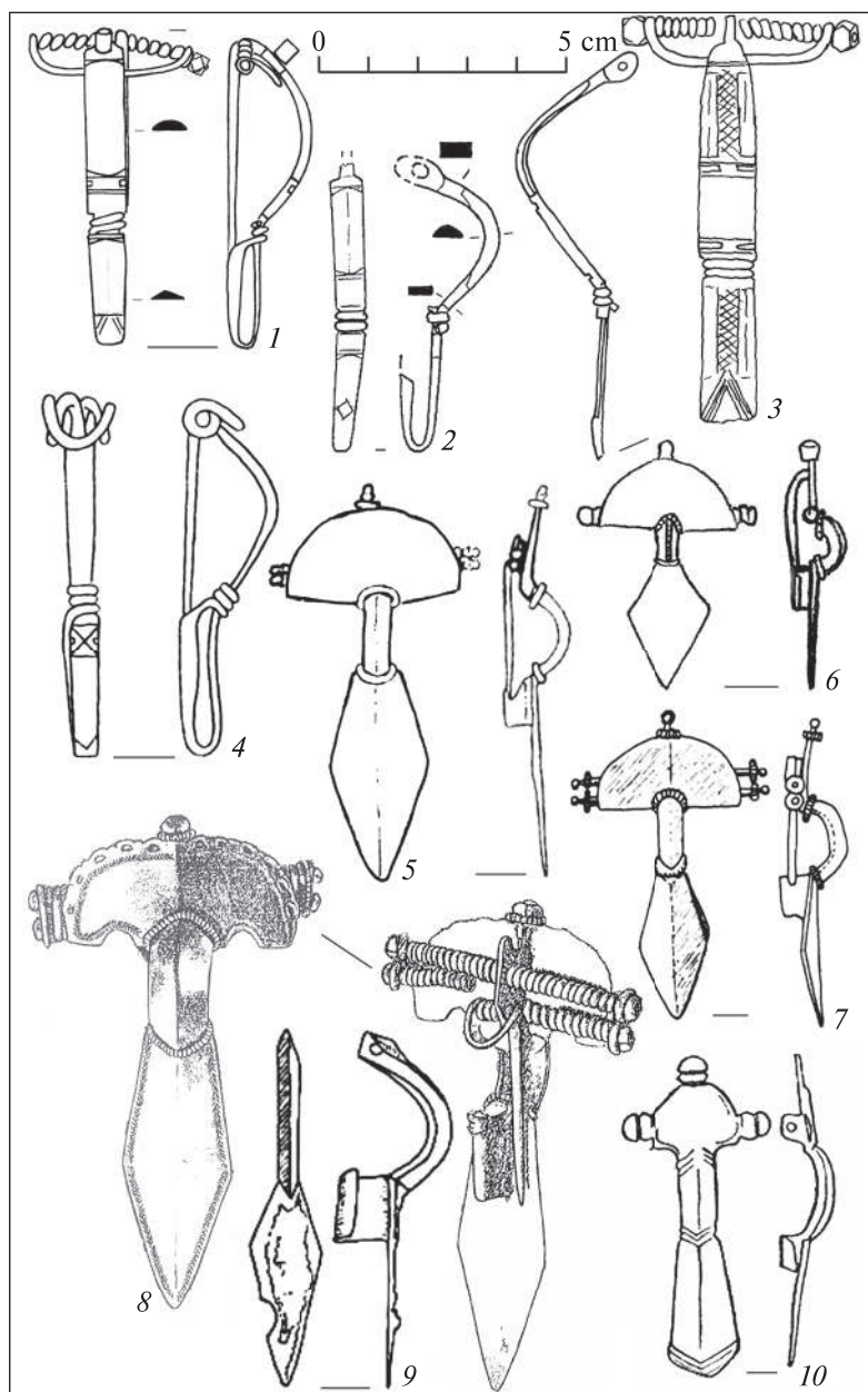
Рис. 5. Фібули пізнього етапу черняхівської культури: 1 — Косанове, к.ш. (Petrauskas 2003, s. 224—351); 2 — Велика Бугаївка / пох. 94 (Петраускас, Шишкин 2013, рис. 124); 3 — Гаврилівка / пох. 5 (Сымонович 1955, с. 282—316); 4 — Баїв / пох. (Кухаренко 1975, рис. 3); 5 — Курники / пох. 4 (Магомедов 1999, рис. 6); 6, 7 — Журавка Вільшанська / пох. 14 (Гавритухин 2007, рис. 10: 1; Гороховский 1988, № 81); 8 — Ранжеве / пох. 14 (Сымонович 1979, с. 93—111); 9 — Київ (Каргер 1948, с. 250—251); 10 — Теремці / житло 14 (Баран 2008, табл. 29: 20)
