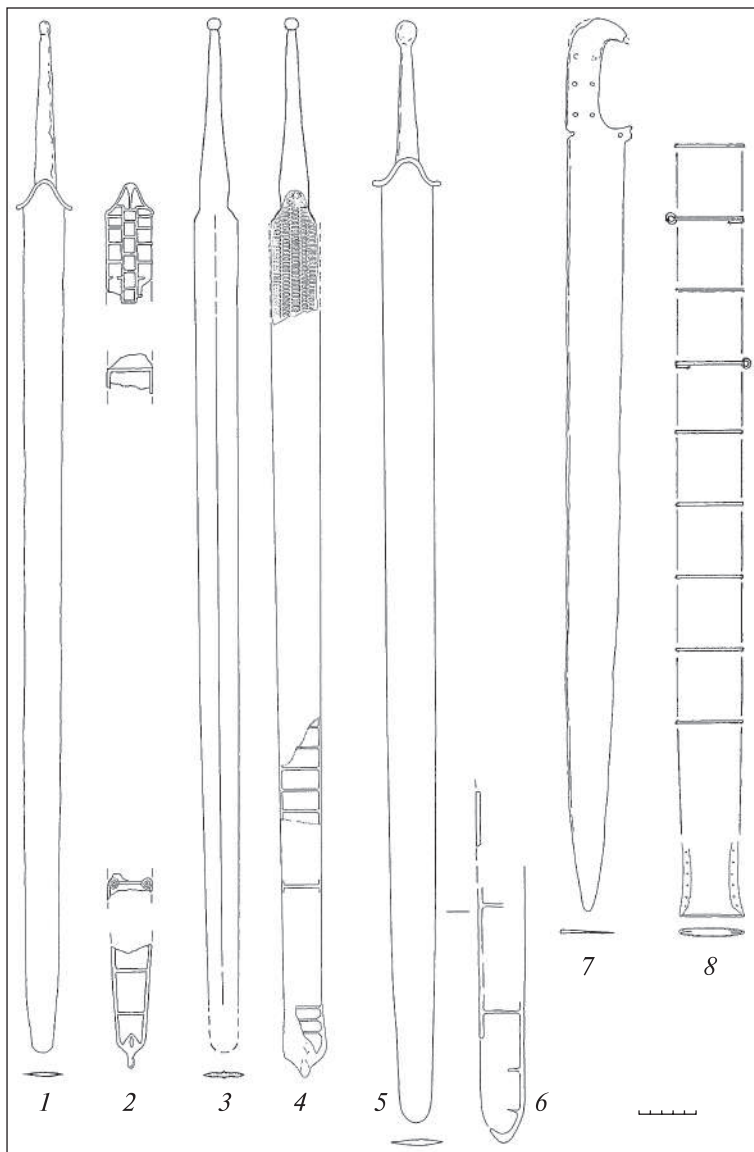
Рис. 3. Мутин. Залізні мечі та піхви: 1, 2, 7, 8 — поховання 8А; 3, 4 — поховання 3; 5, 6 — поховання 7. Рисунки Р. В. Терпиловського та І. М. Ігнатенка
