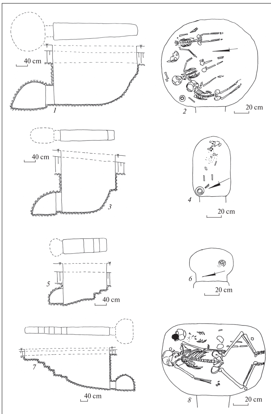
Рис. 1. Катакомби Верхньо-Салтівського-IV могильника (ВСМ-IV). 1, 2 — катакомба 28; 3, 4 — катакомба 32; 5, 6 — катакомба 34; 7, 8 — катакомба 50
