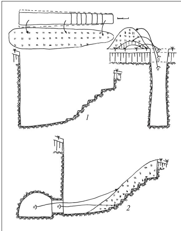
Рис. 4. Схема процесу спорудження катакомби: 1 — послідовність виймання шарів ґрунту з дромосу; 2 — розміщення ґрунту, що виймався при створенні поховальної камери. а — дерен; б — чорнозем, в — материкова глина
