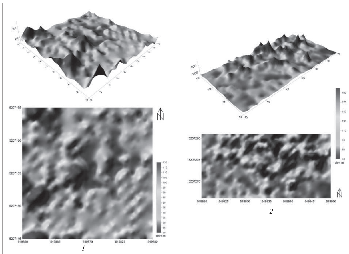
Рис. 8. 1 — распределение удельного сопротивления грунта в диапазоне 50—120 Ом-м для участка E4, В. Малковский; 2 — распределение удельного сопротивления грунта в диапазоне 50—200 Ом-м для участка E5, В. Малковский
