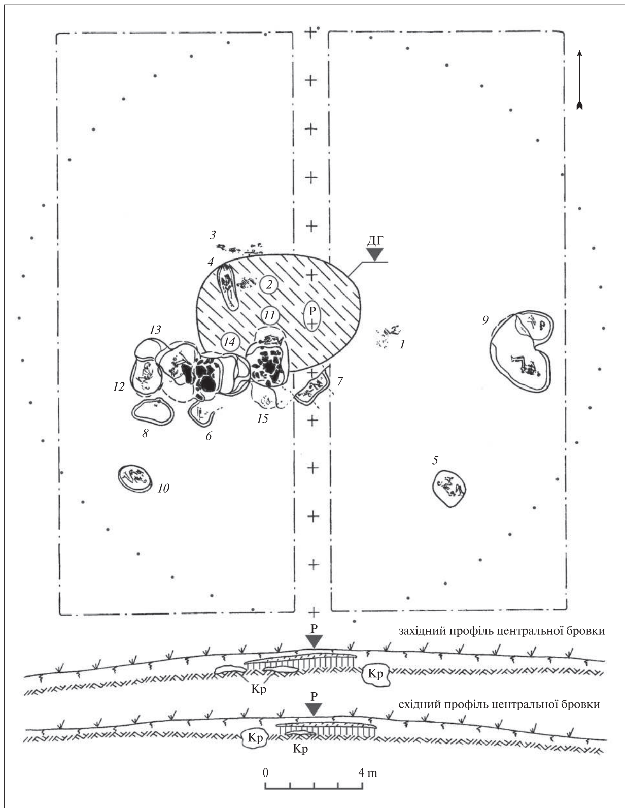
Рис. 2. Загальний план та профілі кургану 1
