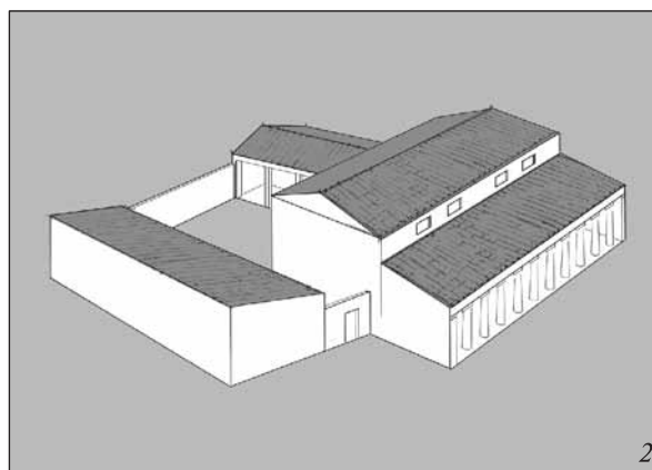
▲ Рис. 7. Ольвія. Загальний вигляд комплексу дикастерія з південного сходу. Реконструкція: 1 — варіант з розміщенням входу в західний і південний блоки в створі з колонадою східного блоку; 2 — те саме в створі з тильною стороною східного портика
