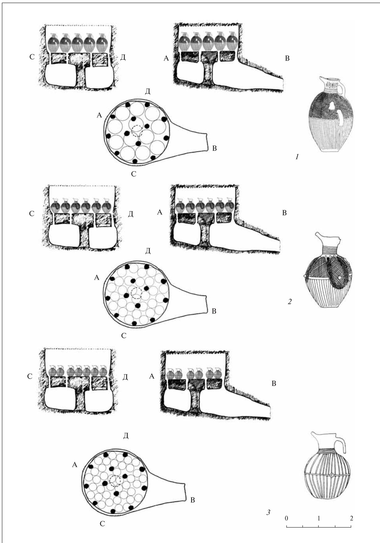
Рис. 4. Моделі розташування посуду в горні: 1 — варіант 1а; 2 — варіант 1б; 3 — варіант 1в (за: Сміленко 1975)
