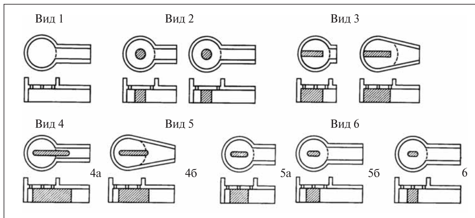
Рис. 3. Схема розподілу горнів на види (за: Бобринский 1991)
