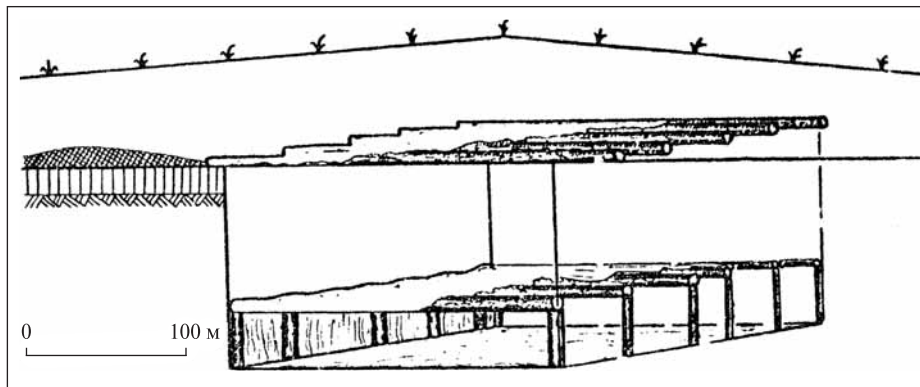
Рис. 3. Реконструкція поховальної споруди в кургані 3 Південного некрополя біля с. Прибузьке
