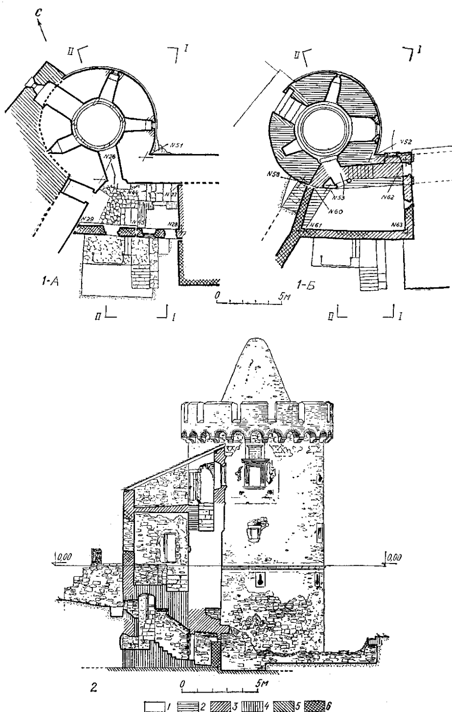
Рис. 6. Плани та фасад башти Рожанки Кам'янець-Подільського замку:
