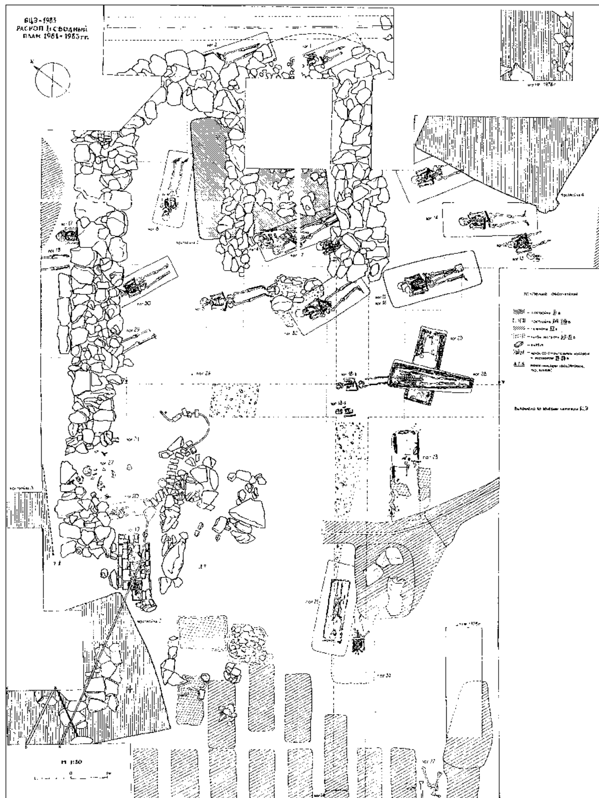
Рис. 1. План фундаменту давньоруського храму за Р.С. Орловим.
