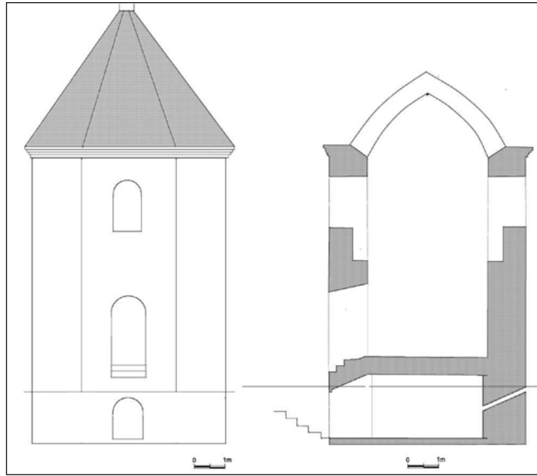
Рис. 2. План східного фасаду та розріз вежі-дзвіниці в с. Суличівка. Обміри О. Бондаря.
