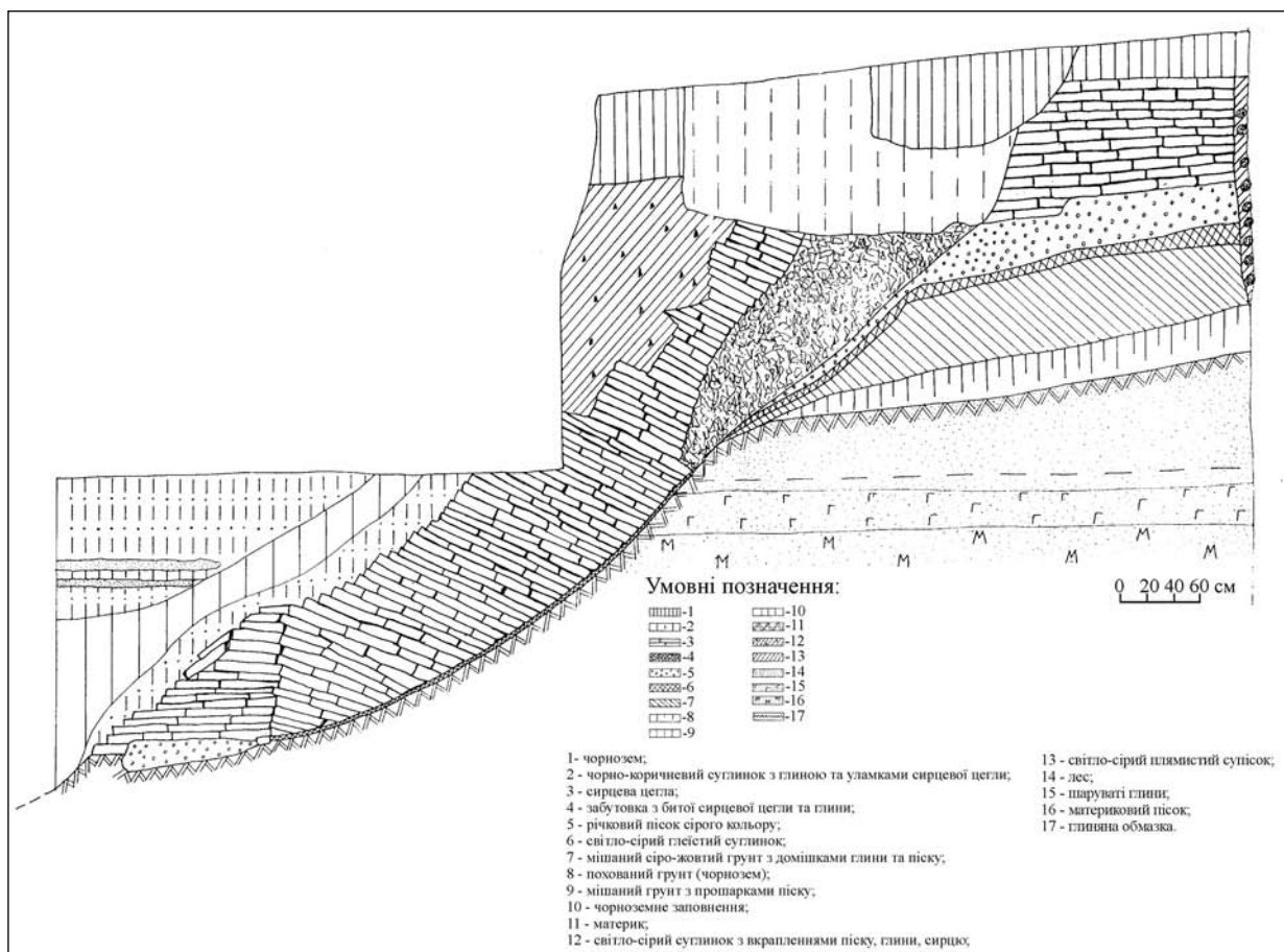
Рис. Перетин сирцевої кладки перед оборонним валом дитинця Переяславля Руського
